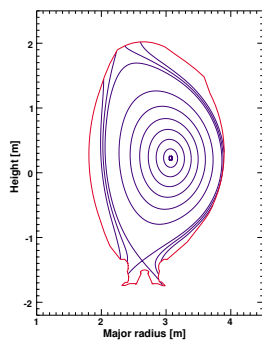
Fig. 4 EHT magnetic configuration
