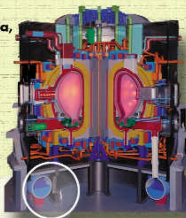
Modelo do ITER (versão de Fevereiro de 1998)
